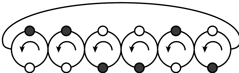
Рис. 2. Бинарная цепочка, N = 6 , левоприоритетное правило разрешения конфликта.
