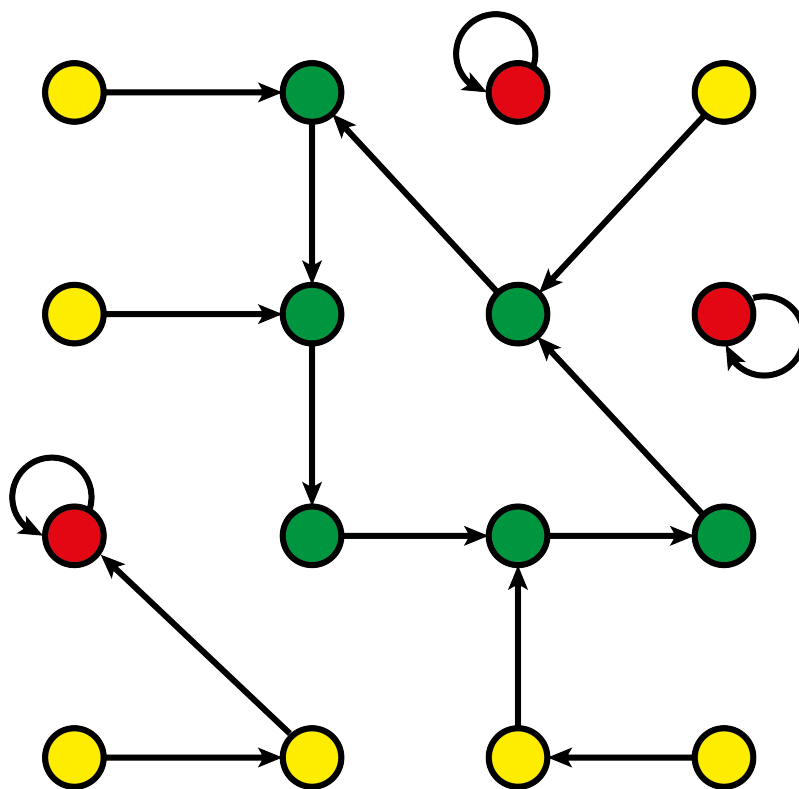
Рис. 1. Возвратные и невозвратные состояния
