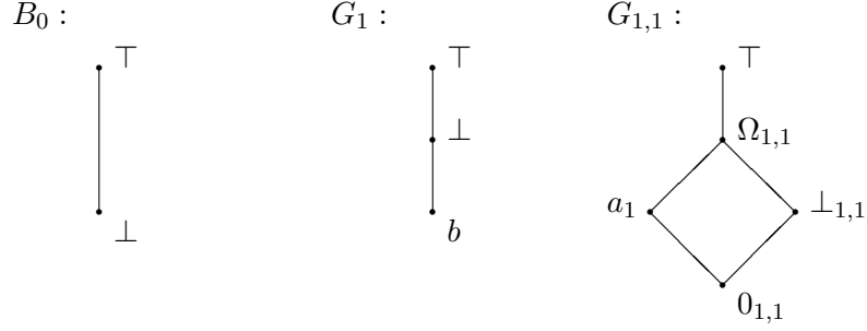
Рис. 1. Алгебры B_0 , G_1 и G_{1,1}
