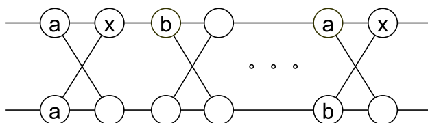
Рис. 13. Недизъюнктные блоки \begin{pmatrix} a \\ a \end{pmatrix} и \begin{pmatrix} a \\ b \end{pmatrix} на расстоянии \rho > 2 , п. б)
