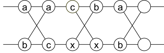
РИС. 6. Недизъюнктивные блоки \begin{pmatrix} a \\ b \end{pmatrix} и \begin{pmatrix} a \\ c \end{pmatrix} в одном 4-цикле
