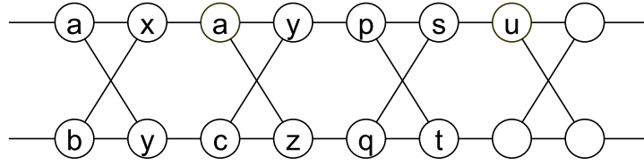
Рис. 10. Недизъюнктные блоки \begin{pmatrix} a \\ b \end{pmatrix} и \begin{pmatrix} a \\ c \end{pmatrix} на расстоянии \rho = 2
