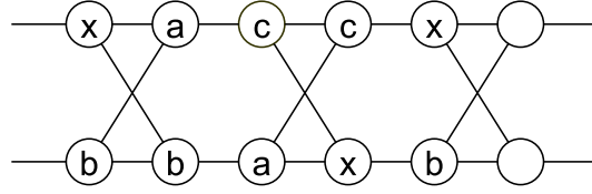
Рис. 7. Недизъюнктные блоки \begin{pmatrix} a \\ b \end{pmatrix} и \begin{pmatrix} c \\ a \end{pmatrix} в одном комплексе
