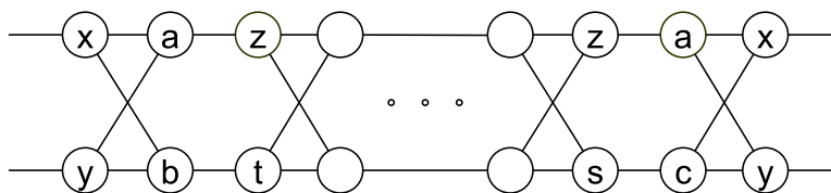
Рис. 14. Недизъюнктные блоки \begin{pmatrix} a \\ b \end{pmatrix} и \begin{pmatrix} a \\ c \end{pmatrix} на расстоянии \rho > 2 , п. а)
