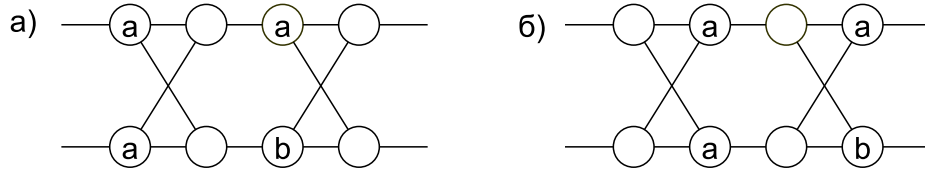
Рис. 8. Недизъюнктные блоки \begin{pmatrix} a \\ a \end{pmatrix} и \begin{pmatrix} a \\ b \end{pmatrix} на расстоянии \rho = 2
