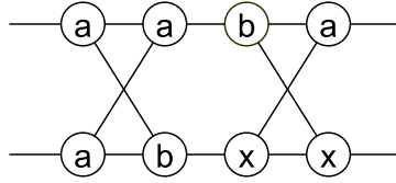
Рис. 5. Недизъюнктивные блоки \begin{pmatrix} a \\ a \end{pmatrix} и \begin{pmatrix} a \\ b \end{pmatrix} на расстоянии \rho = 1
