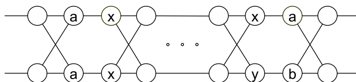
Рис. 12. Недизъюнктные блоки \begin{pmatrix} a \\ a \end{pmatrix} и \begin{pmatrix} a \\ b \end{pmatrix} на расстоянии \rho > 2 , п. а)
