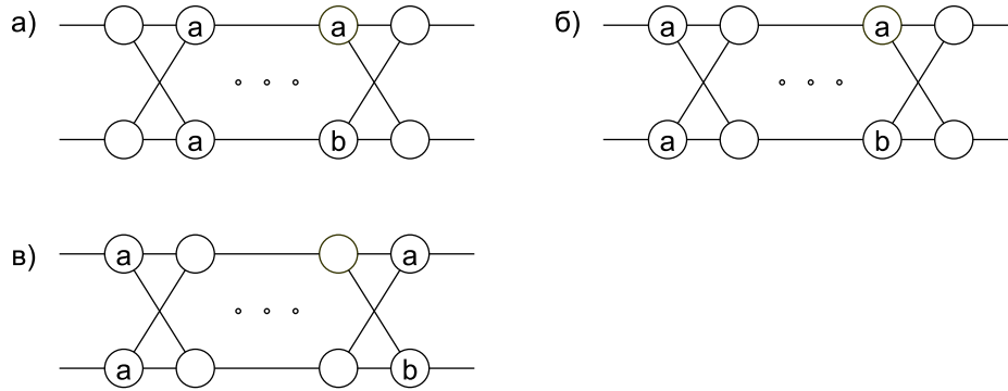
Рис. 11. Недизъюнктные блоки \begin{pmatrix} a \\ a \end{pmatrix} и \begin{pmatrix} a \\ b \end{pmatrix} на расстоянии \rho > 2
