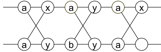
Рис. 9. Недизъюнктные блоки \begin{pmatrix} a \\ a \end{pmatrix} и \begin{pmatrix} a \\ b \end{pmatrix} на расстоянии \rho = 2 , п. а)
