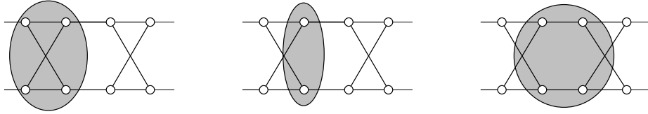
Рис. 2. 4-цикл, блок и комплекс скрещенной призмы
