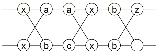
Рис. 4. Доказательство леммы 3
